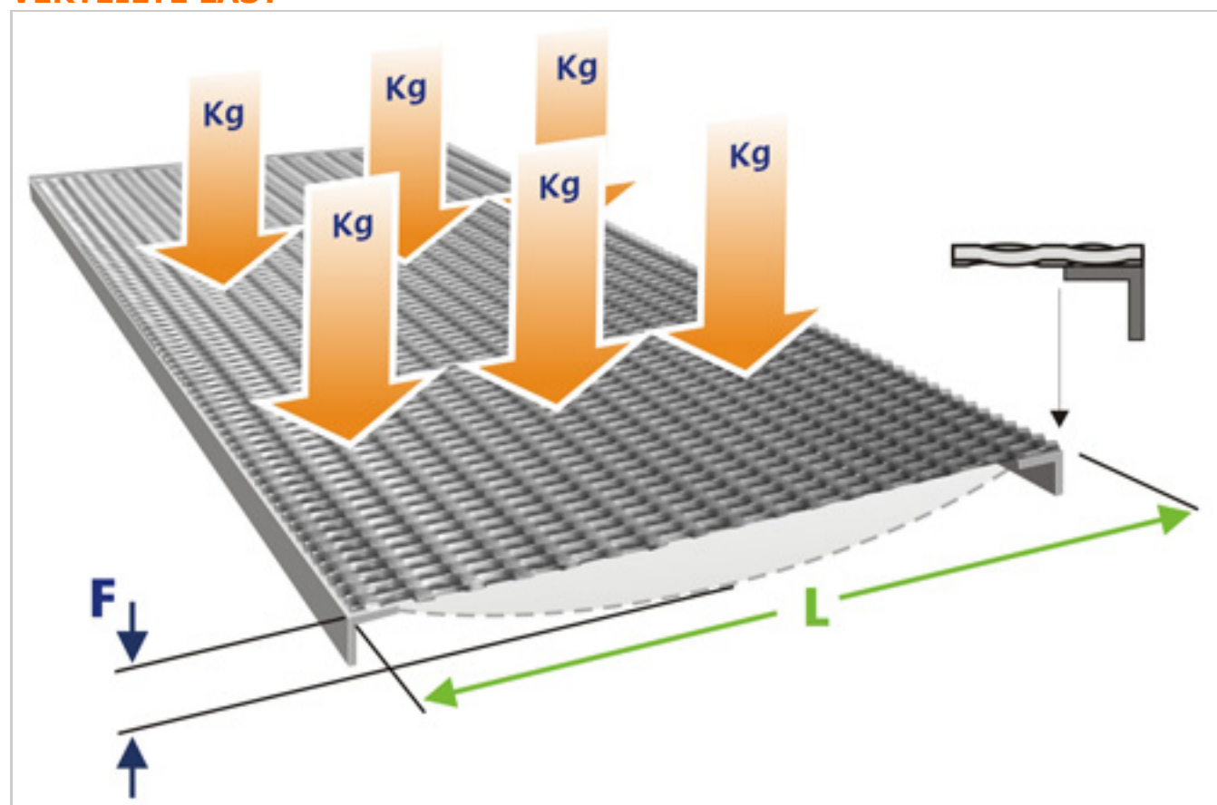
F DURCHBIEGUNG - L SPANNWEITE
