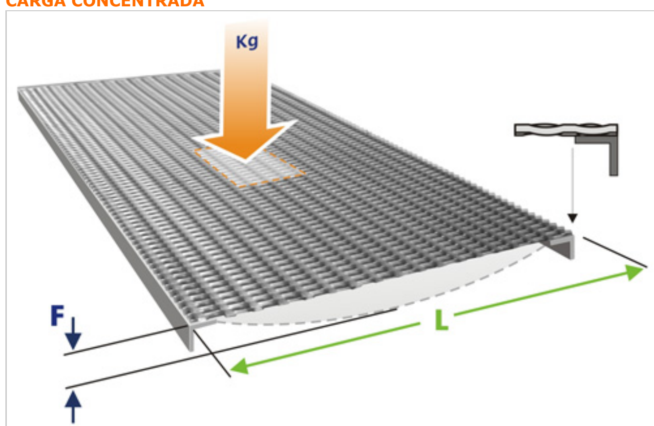
F FLECHA DE INFLEXION - L LUZ LIBRE
