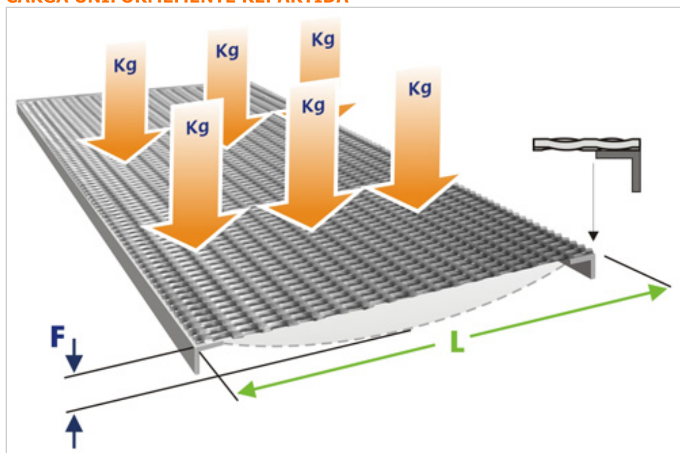
F FLECHA DE INFLEXION - L LUZ LIBRE
